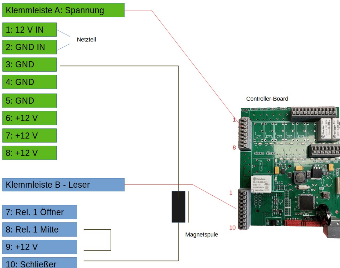
Abbildung 16: dauerstrombetriebener Türöffner
