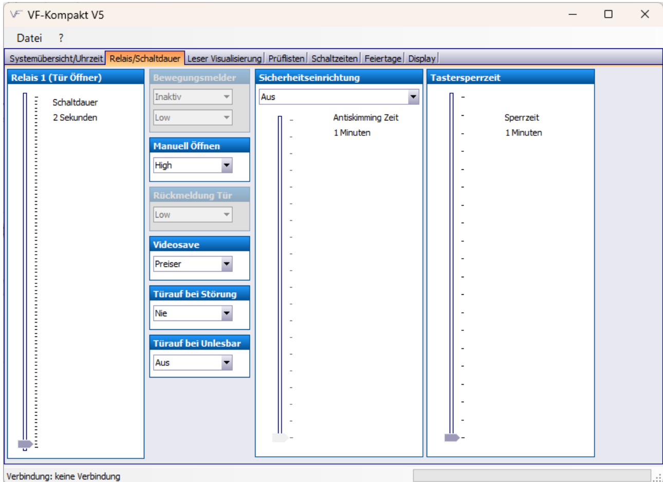
Abbildung 19: Übersicht Relais/Schaltdauer
