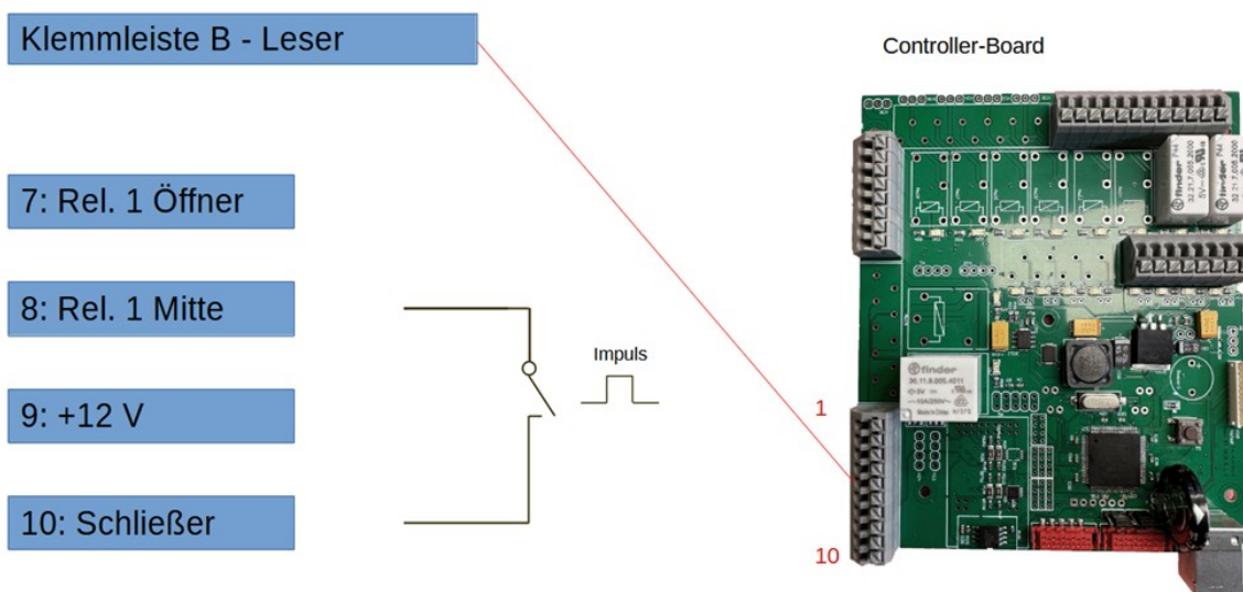
Abbildung 15: Anschluss impulsgesteuerter Türöffner
